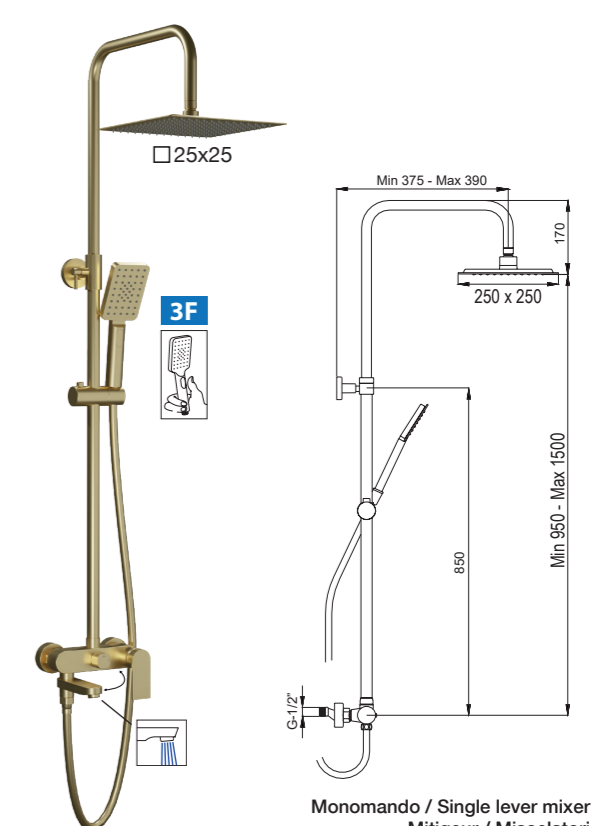
Monomando / Single lever mixer Mitigeur / Miscelatori 21NITC25ASB09 XXX,XX€ 6024X2 9 l/min 3 bar +4,80€
